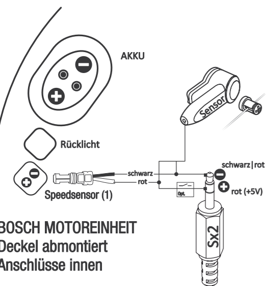
Abbildung Klemmraum Motor
