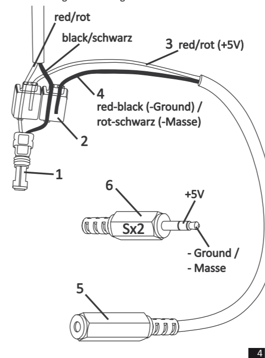
Abbildung Bezeichnungen Sx2KB Bosch Classic Kabelkit
